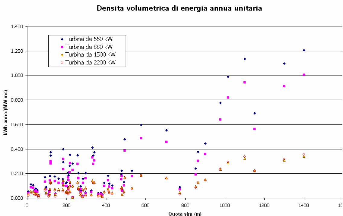
Fig. 4.14 – Densità volumetrica di energia annua prodotta
