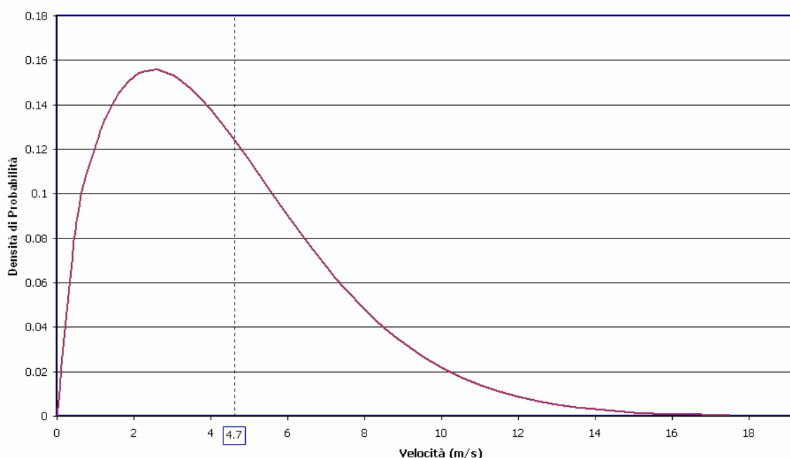
Fig. 4.18 - Distribuzione di Weibull per siti offshore in prossimità della costa marchigiana
