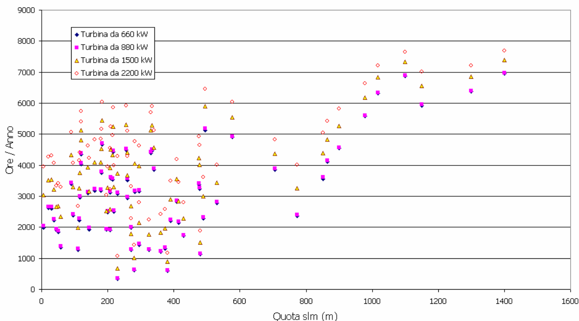
Fig. 4.10 – Ore annue di possibile funzionamento della turbina
