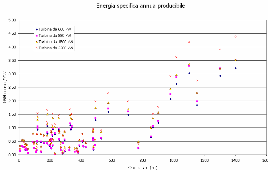
Fig. 4.9 – Energia annua producibile per ogni MW di turbina installato
