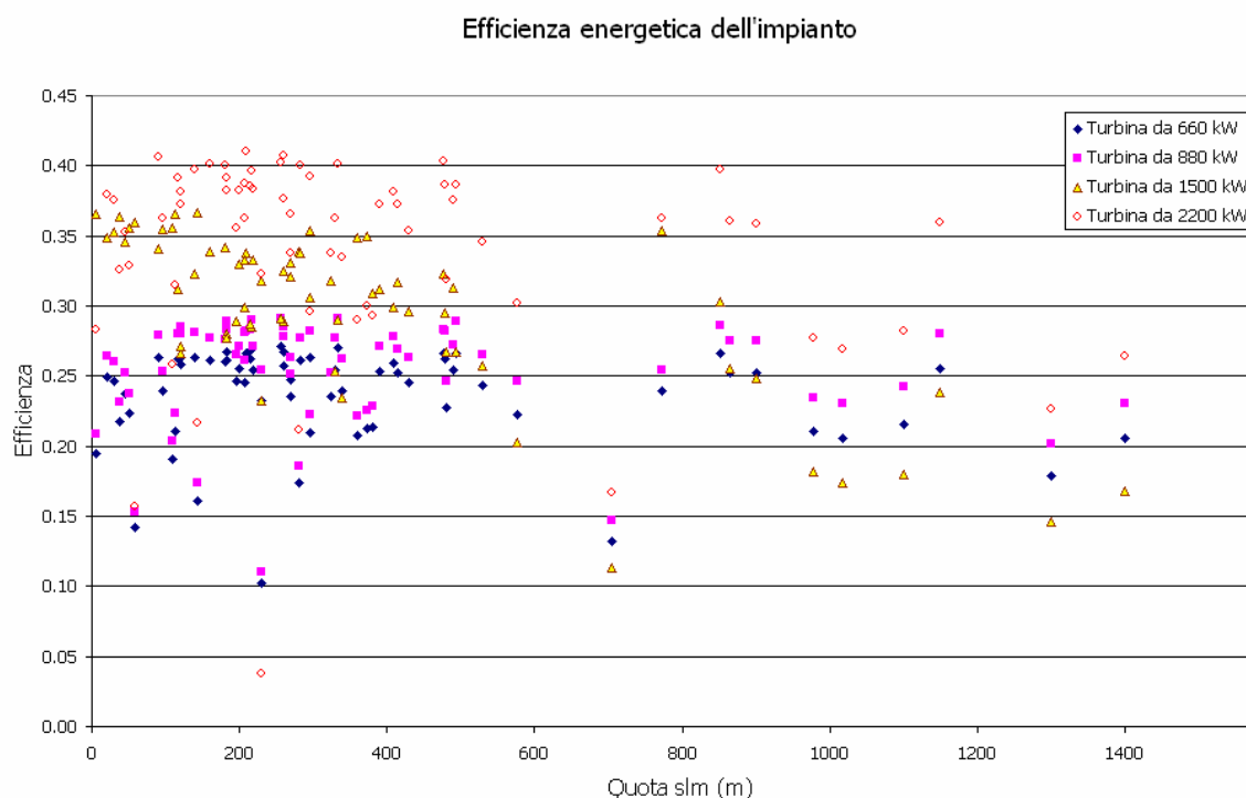
Fig. 4.12 – Efficienza energetica dell'impianto
