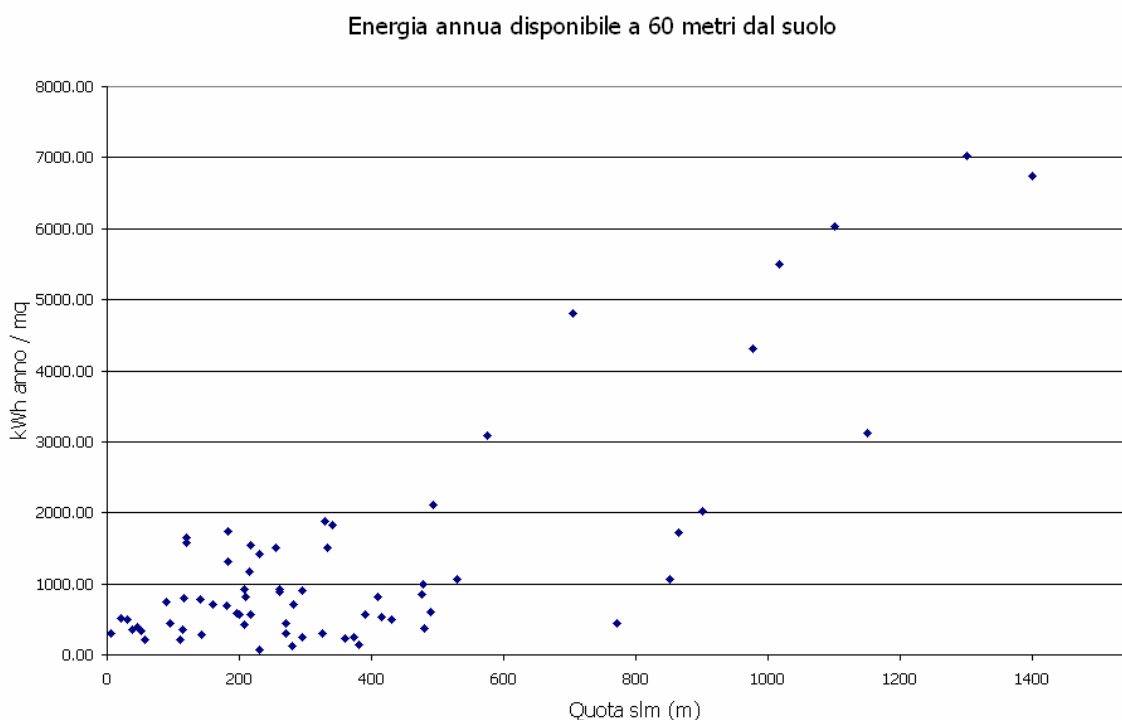
Fig. 4.8 – Energia annua disponibile nei siti marchigiani
