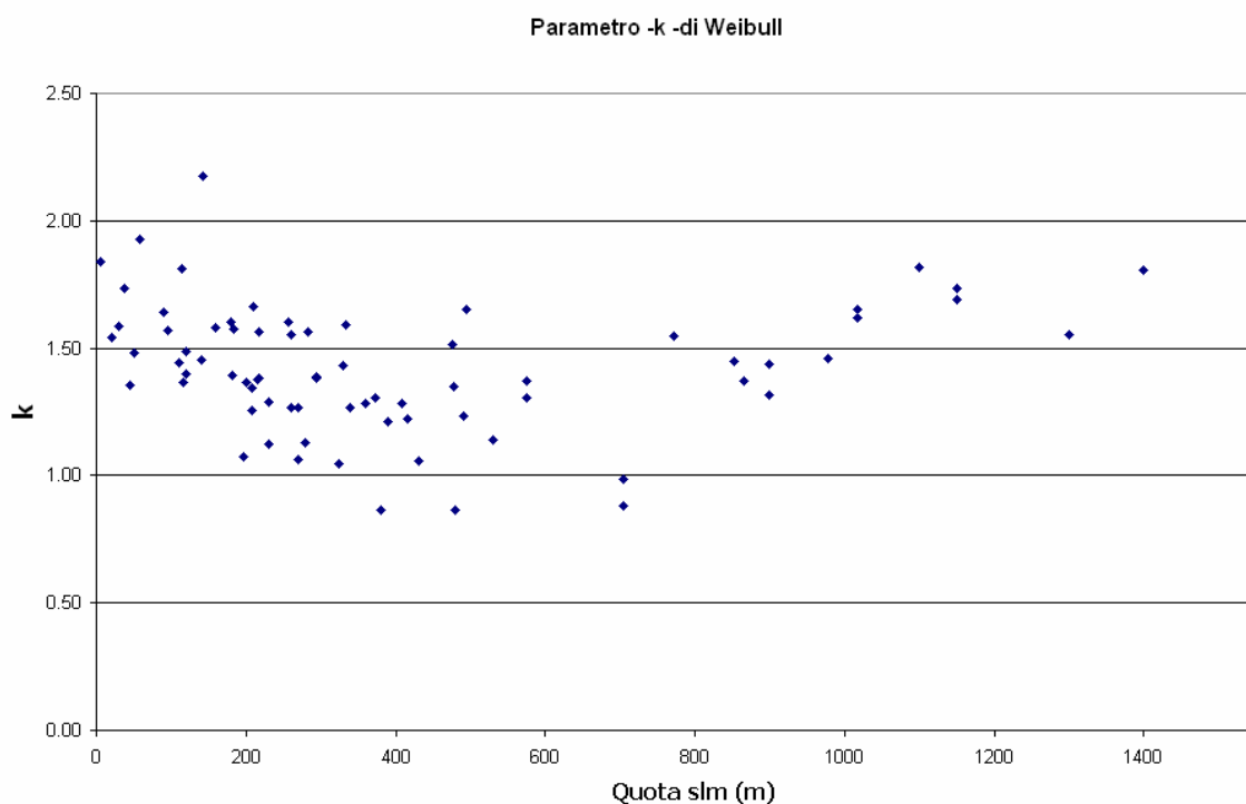
Fig. 4.7 – Andamento di k per varie stazioni meteo site nel territorio marchigiano
