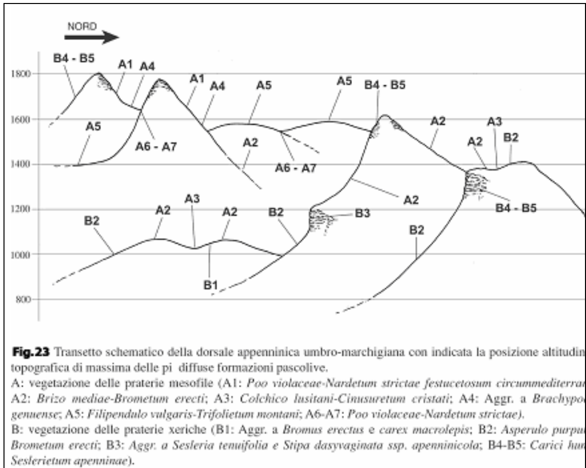
Fig. 4.23 – Transetto schematico della dorsale appenninica umbro-marchigiana
