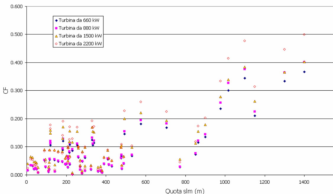
Fig. 4.11 - Fattore di utilizzo dell'impianto eolico
